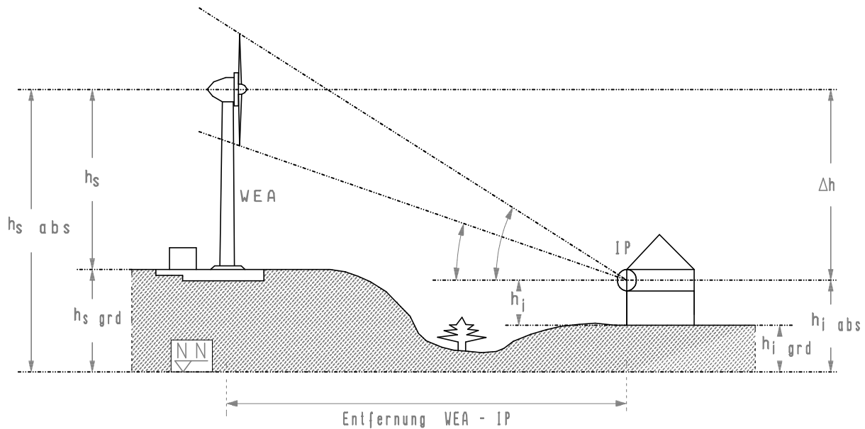
Abb. 3: Geometrische Verhältnisse, Vertikalschnitt
